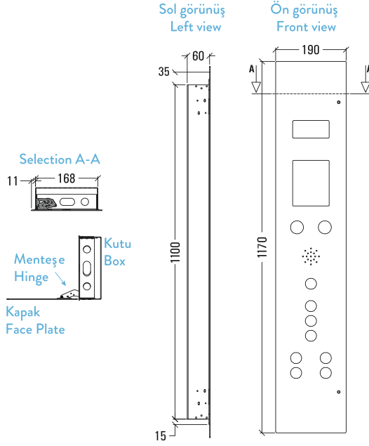
Menteşeli yarım panel / Hinged half C.O.P.
